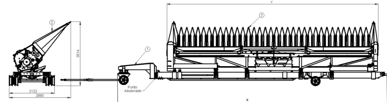
CABEZAL GIRASOLERO CG 2010. Adaptable a cualquier tipo de cosechadora mediante embocador abulonado.
